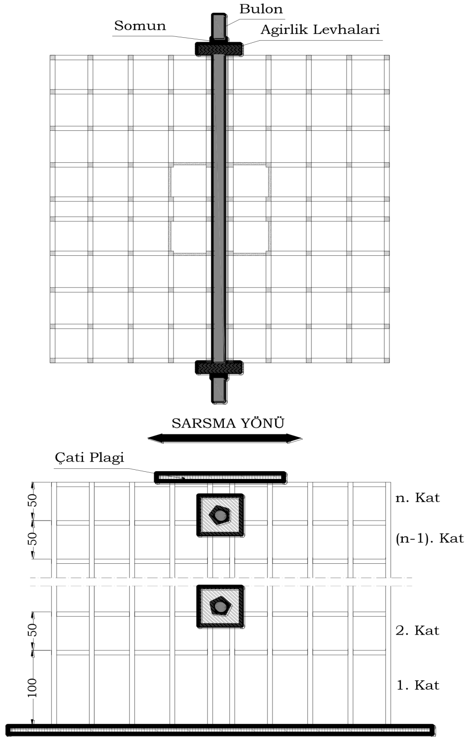
Şekil A6. Kat ağırlıklarının bina maketine yerleşimi: Plan (üst) ve kesit (alt) görünüşleri
