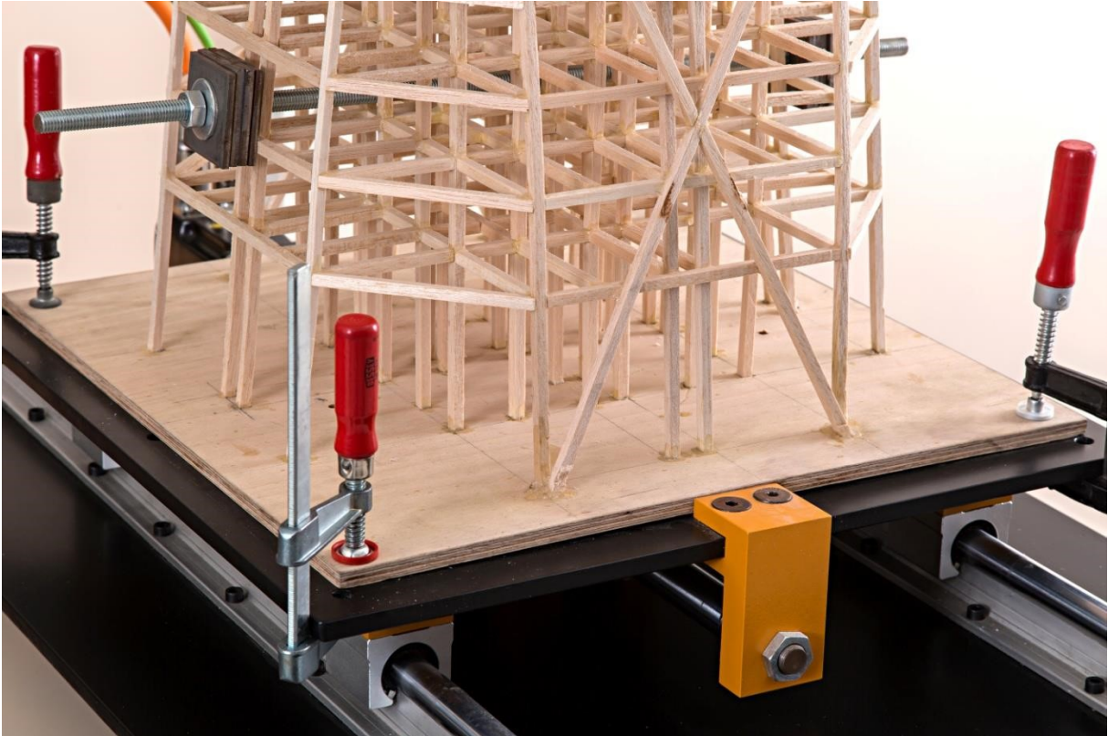
Şekil E10. Mergeneler ile sarsma masasına sabitlenmiş maket ve taban plakası
