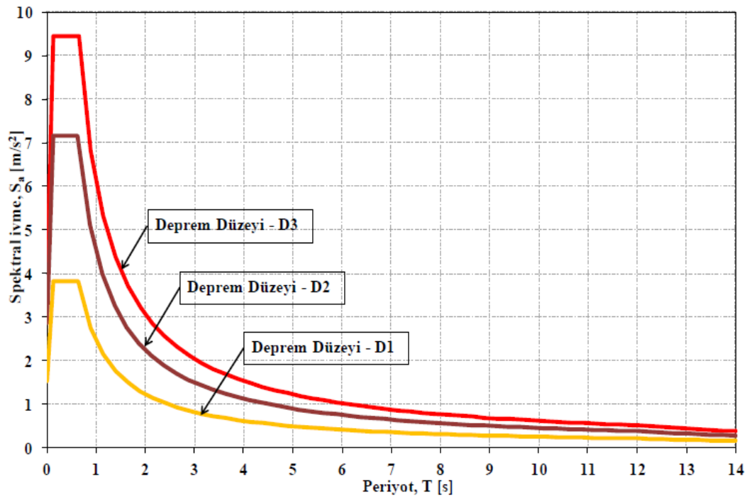
Şekil C1. D1, D2 ve D3 deprem düzeyleri için deprem tasarım spektrumları
