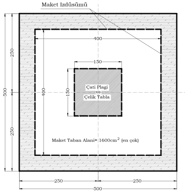
Şekil A3. Taban plakası özellikleri ve yerleşim detayı
