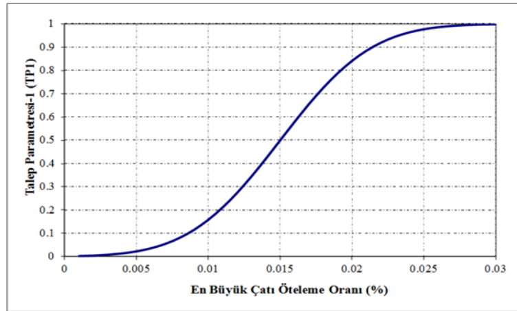
Şekil 6.1. En büyük çatı öteleme oranı ile yapısal hasar kaynaklı kayıp ilişkisini gösteren kayıp fonksiyonu
