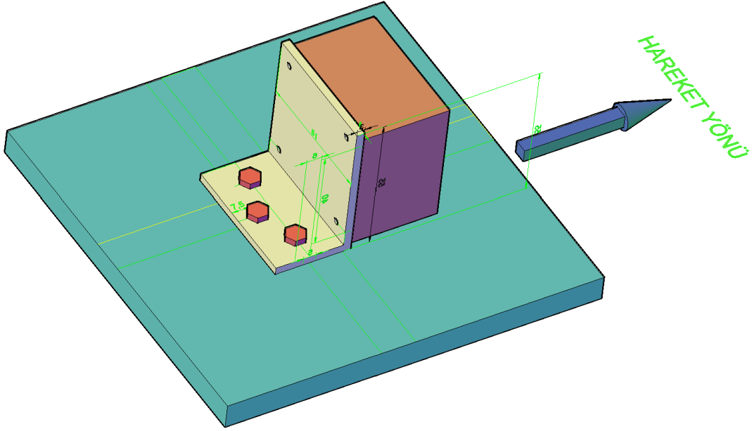
Şekil A1. Maket üzerine yerleştirilmiş ölçüm düzeneğinin genel görünüşü ve metal çatı levhası ve ivmeölçer bağlantısı
