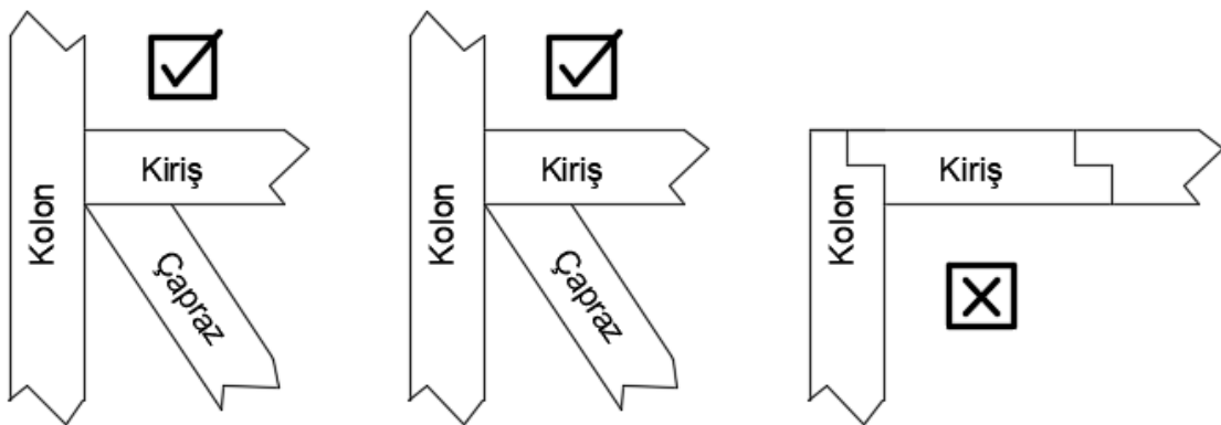
Şekil A7. Guse uygulanmasında izin verilen birleşim ve bağlantı detaylarının düşey kesitte görünüşü
