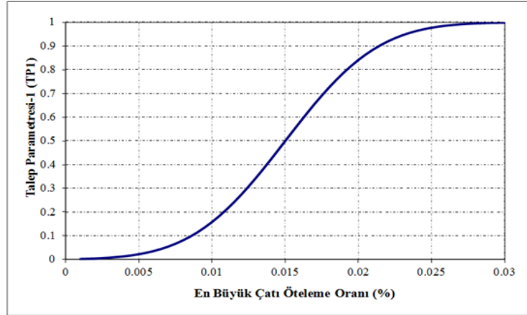
Şekil 6.1. En büyük çatı öteleme oranı ile yapısal hasar kaynaklı kayıp ilişkilendiren kayıp fonksiyonu
