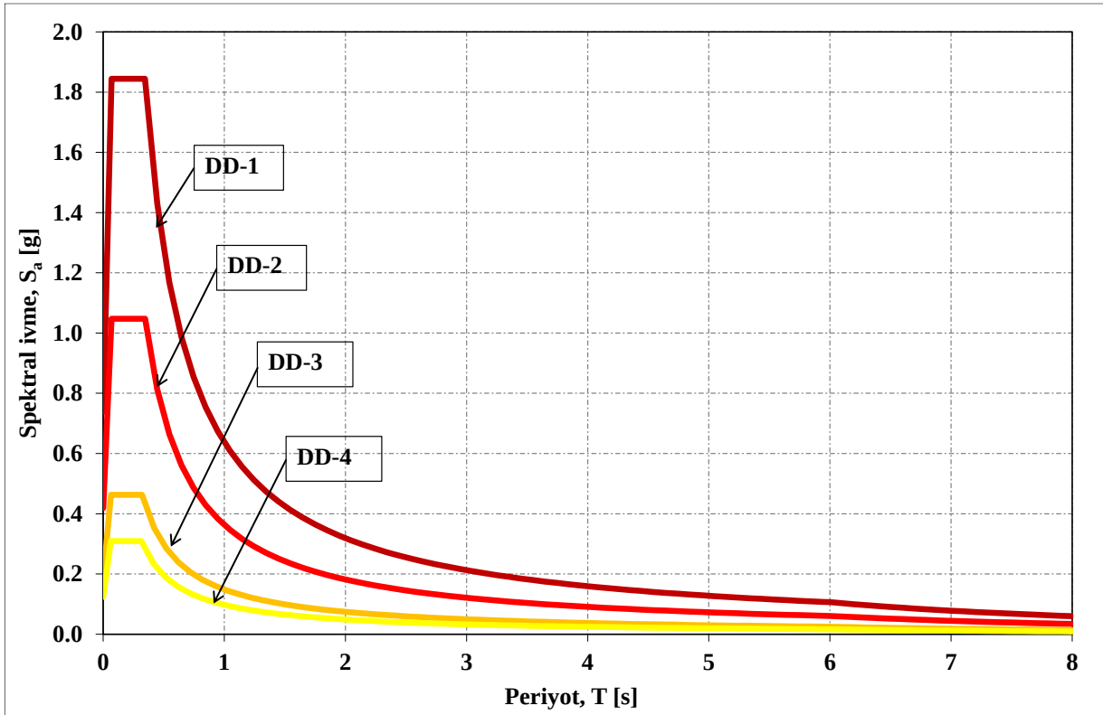
Şekil C1. DD-1, DD-2, DD-3 ve DD-4 deprem düzeyleri için yatay elastik tasarım spektrumları
