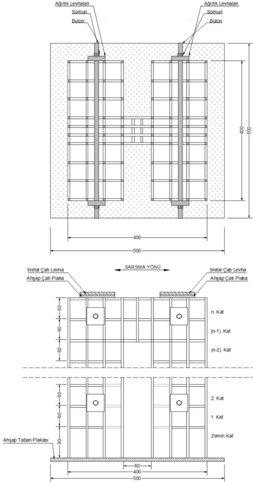
Şekil A.5. Kat ağırlıklarının bina maketine yerleşimi: Plan (üst) ve kesit (alt) görünüşleri
