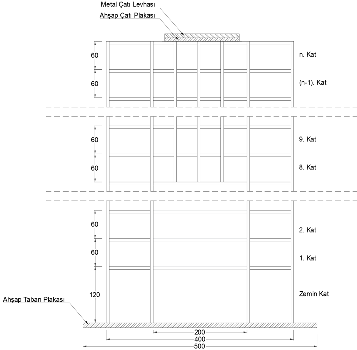
Şekil 2 Bina maketi şematik kesiti
