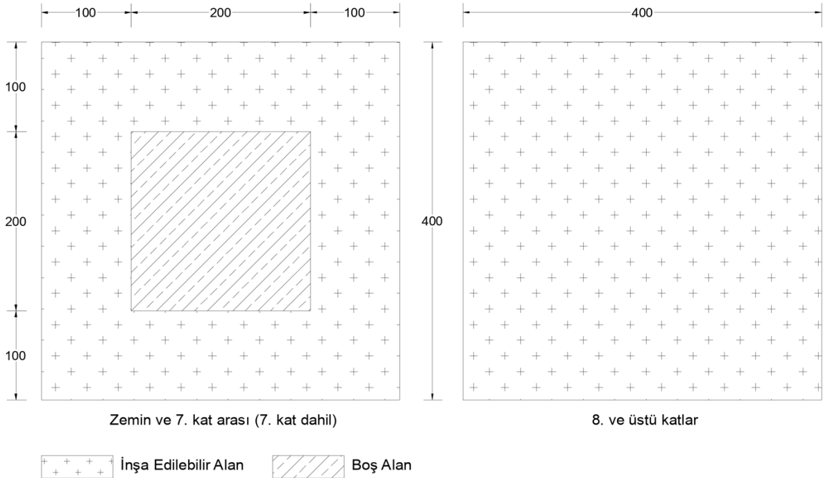
Şekil 1 Bina maketi şematik kat planları
